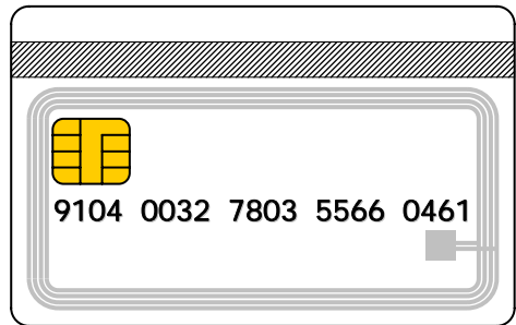
MS付き接触・非接触一体型ICカード(ハイブリッド)
